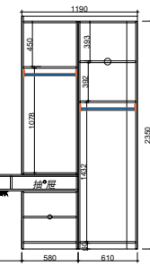
主结构D图
