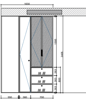
衣柜正视图
