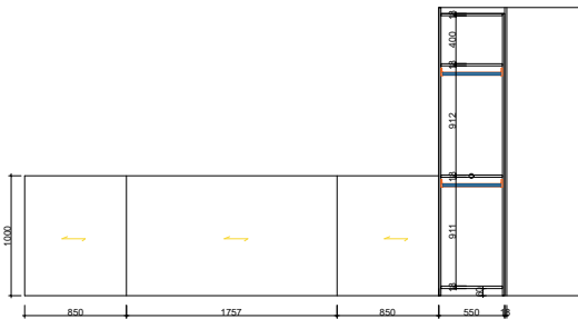
墙板结构图
