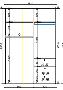
衣柜结构图
