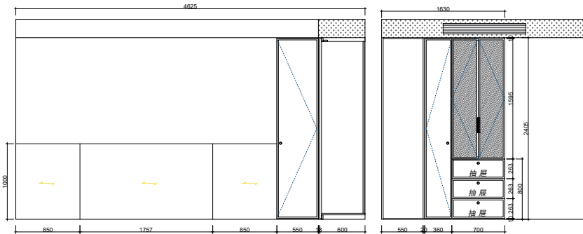
衣柜正视图
