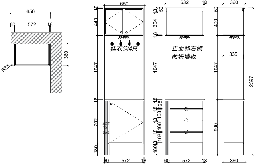
鞋柜正视图
