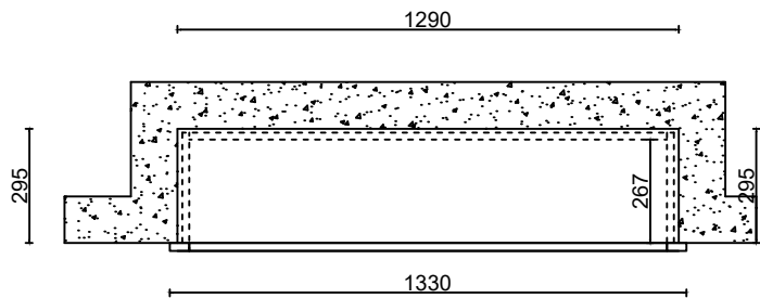
柜体俯视图
