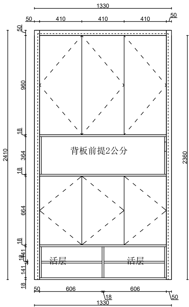
柜体门板图
