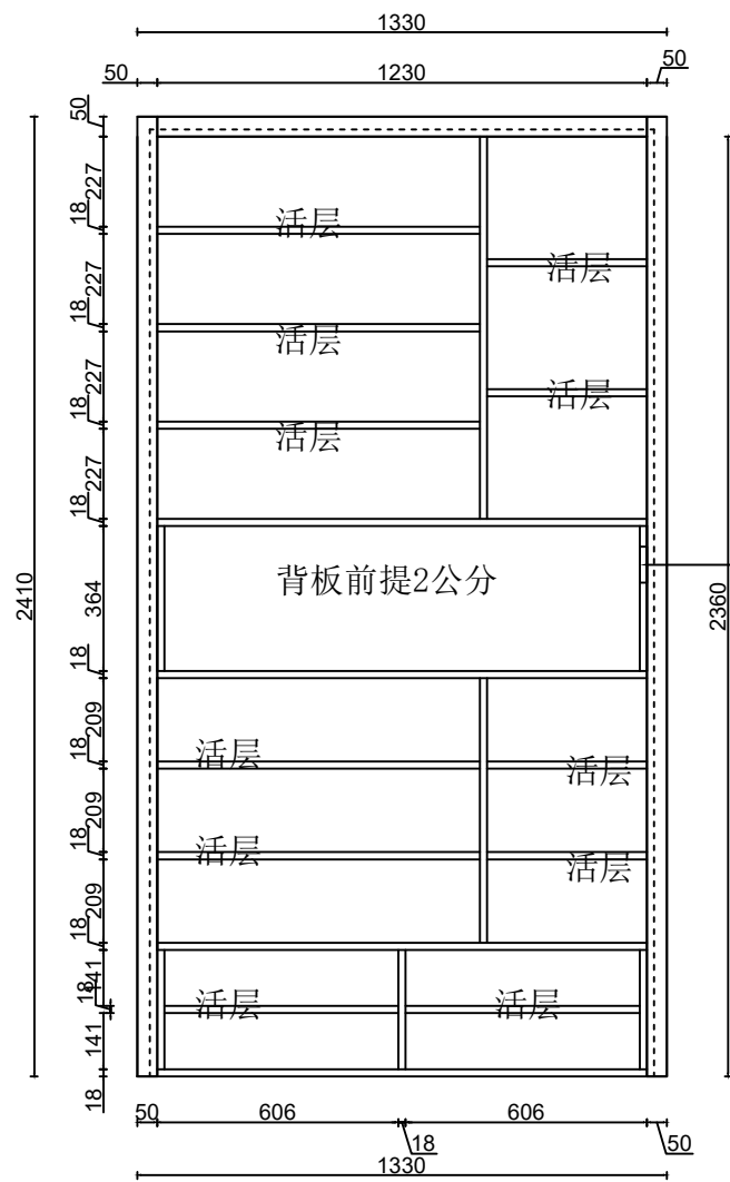
柜体结构图
