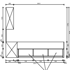
C墙柜体立面图 侧视图
