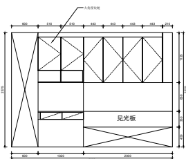
A墙柜体立面图 侧视图
