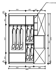
B墙柜体立面图 侧视图
