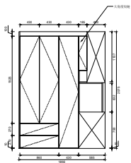
B墙柜体立面图 侧视图
