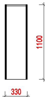
侧视图
