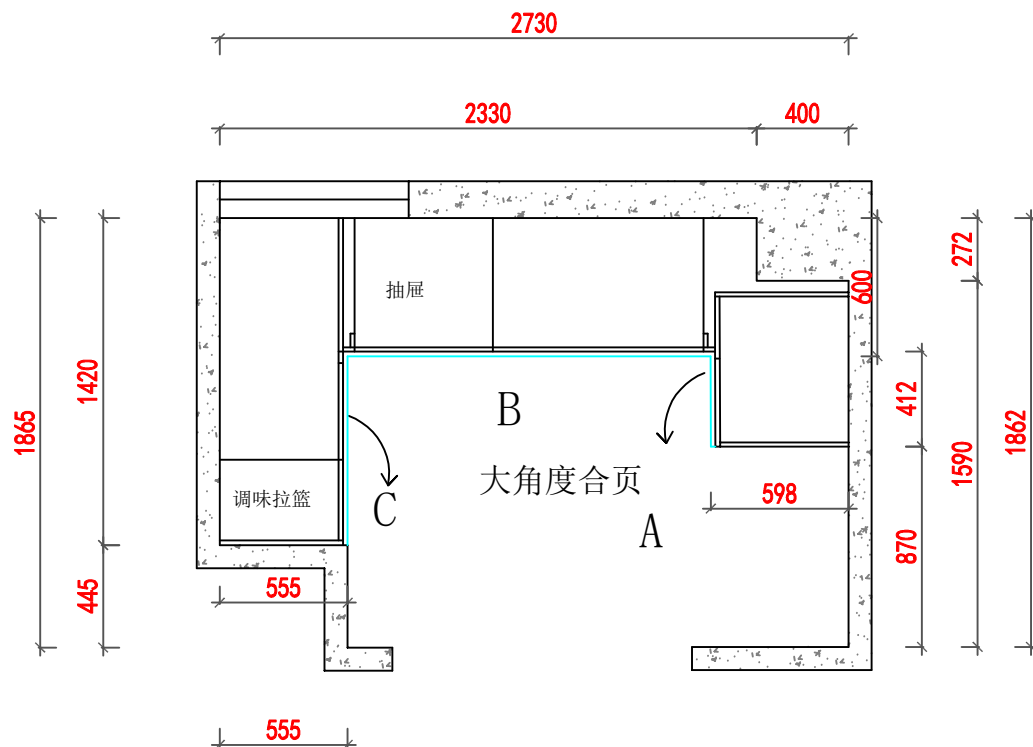
地柜
