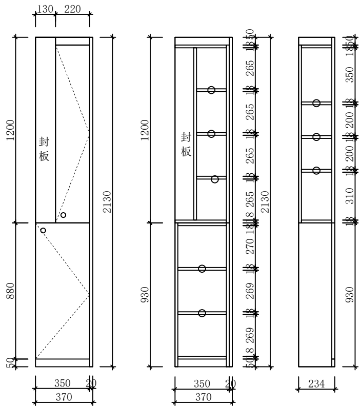
A面门板图 A面柜体图 B面柜体图
